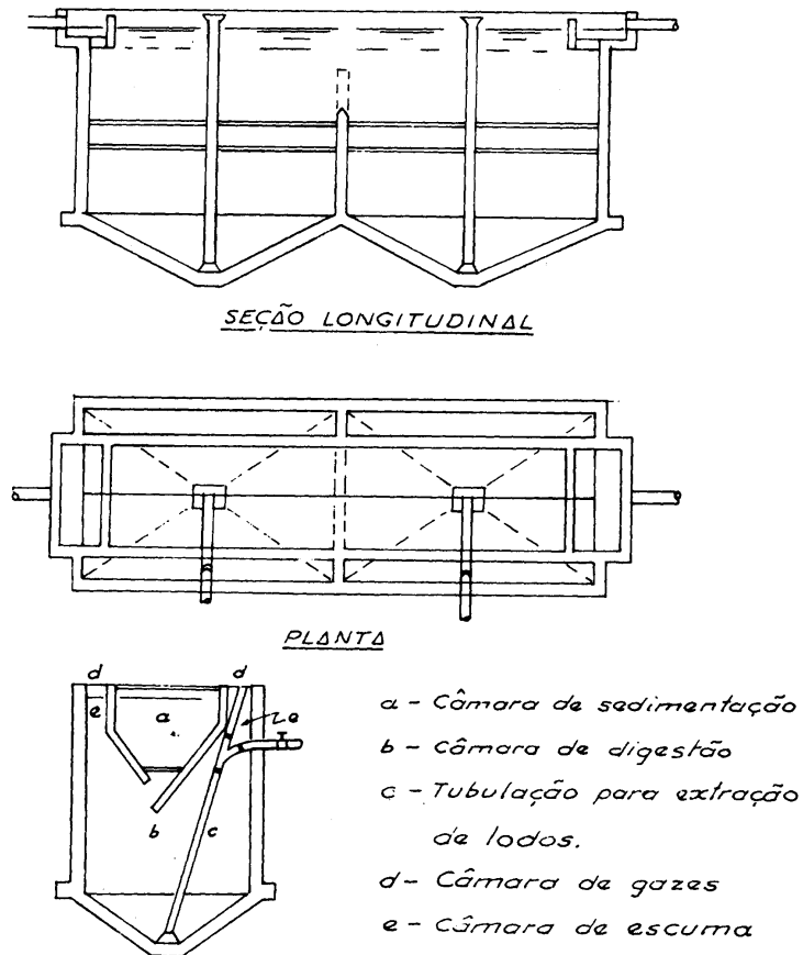
Figura 112 - Tanque Imhoff
