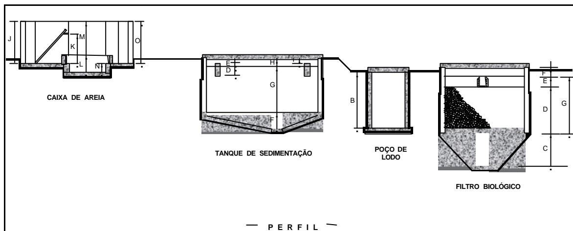
Figura 109 - Perfil da ETE
