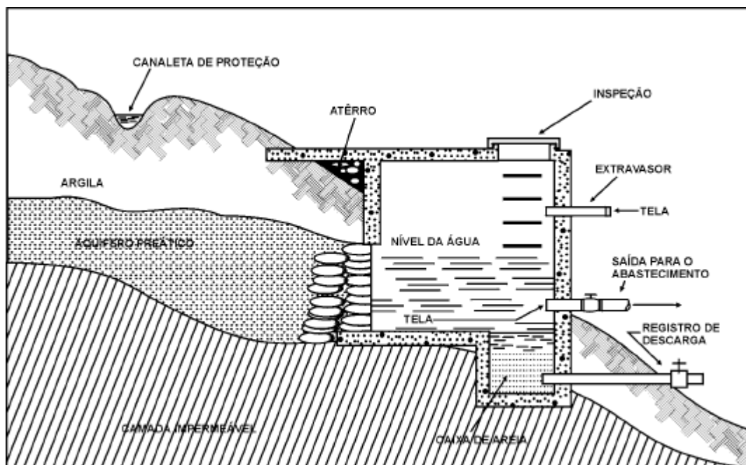
Figura 15 - Caixa de Tomada - Fonte de Encosta
