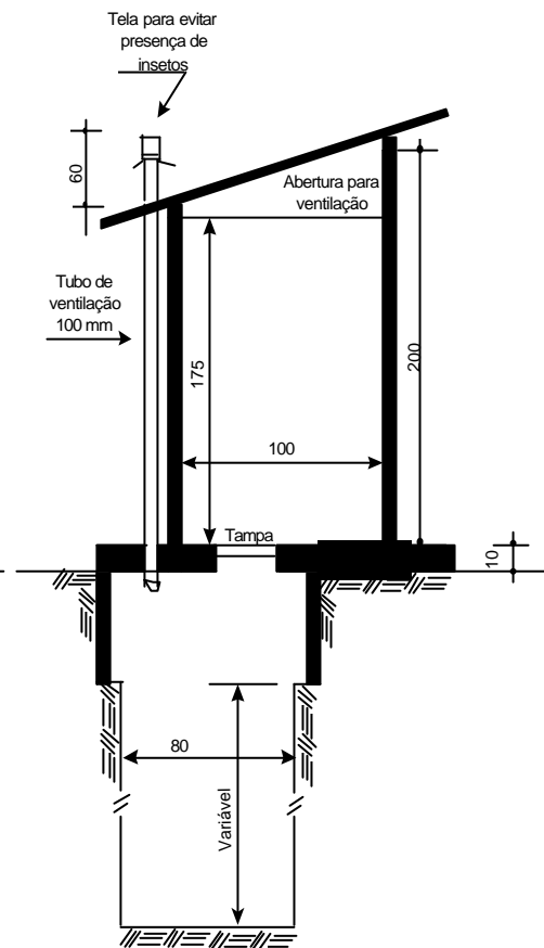
Figura 83 - Privada com Fossa Seca Ventilada
