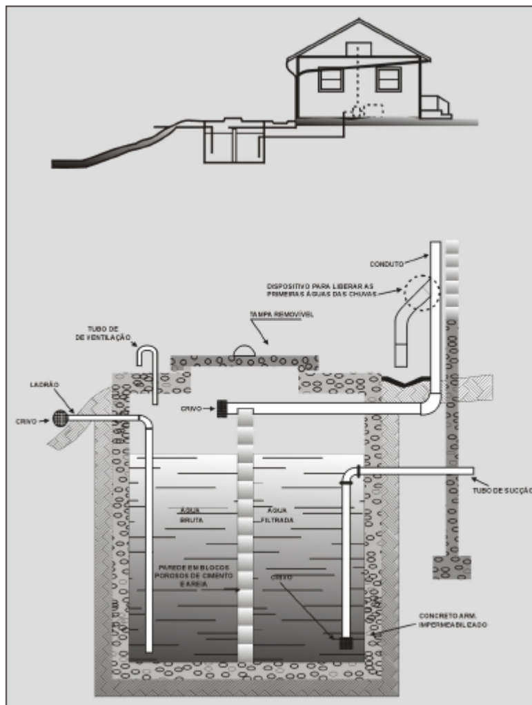
Figura 14 - Corte de uma Cisterna bem Projetada
