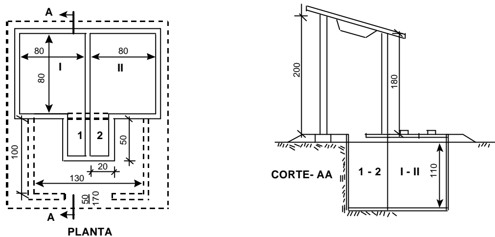
Figura 92 - Privada com Fossa de Fermentação Enterrada
