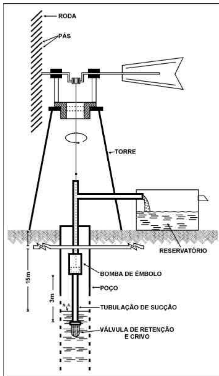
Figura 67 – Esquema de Cata-Vento
