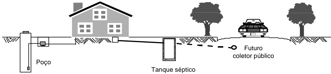
Figura 104 - Esquema de Instalação de Tanque Séptico e Valas de Infiltração
