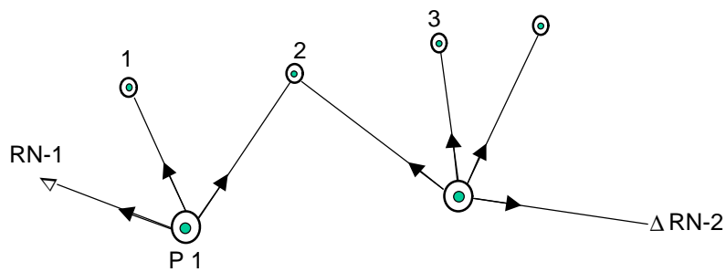
Figura 174 – Nivelamento Irradiado Composto
