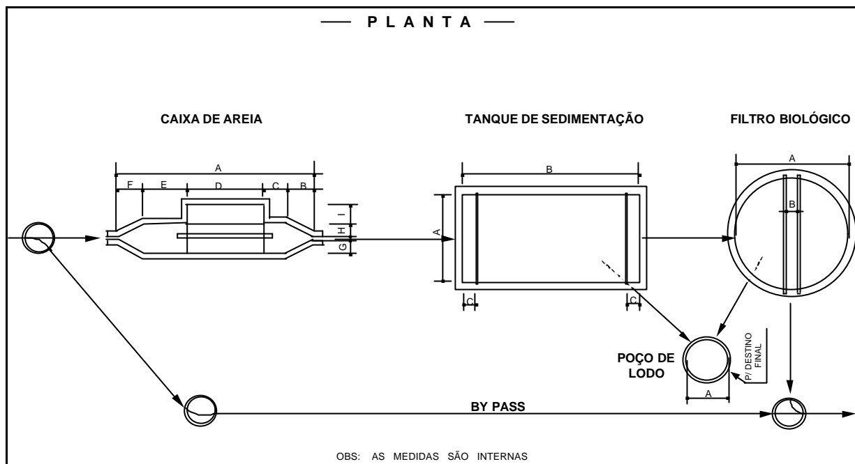
Figura 108 - Planta Baixa de uma ETE
