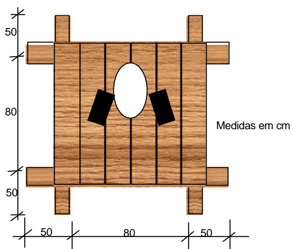
Figura 88 - Base e Piso de Madeira para Privada
