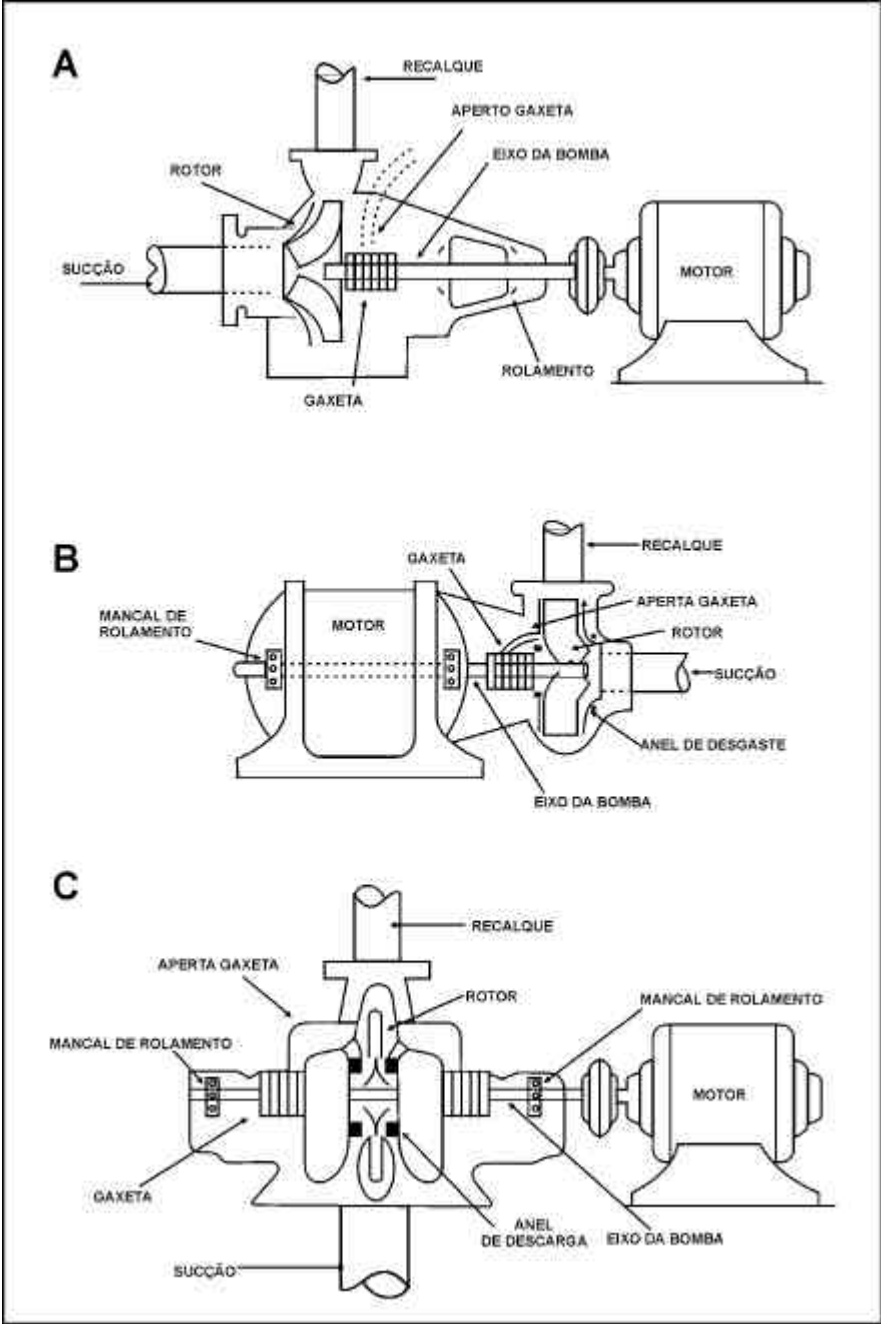
Figura 69 – Bombas Centrífugas
