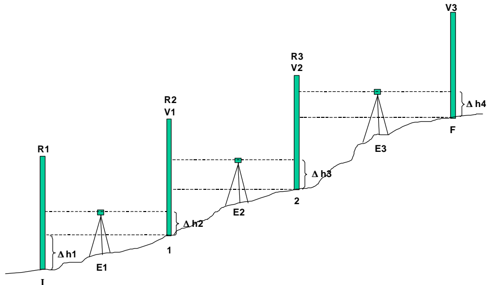
Figura 172 – Nivelamento Linear Composto
