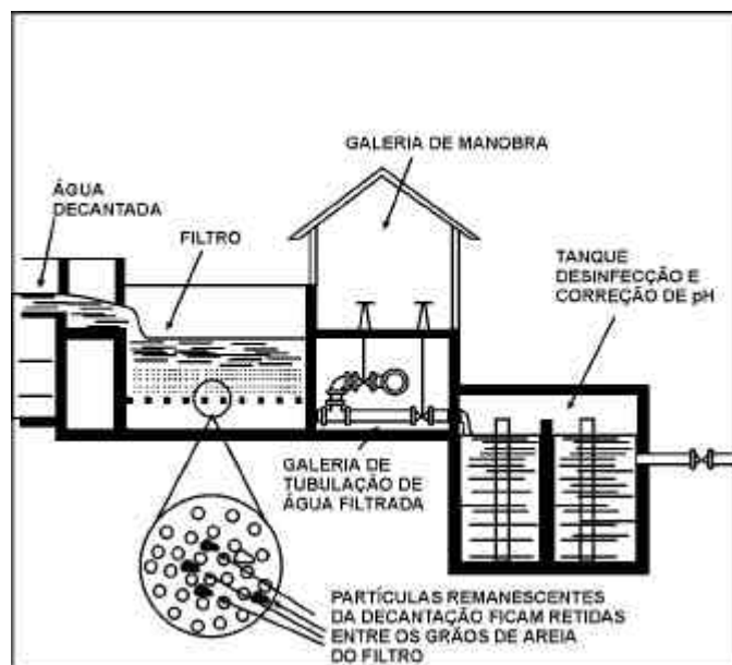
Figura 47 - Filtração Rápida Descendente
