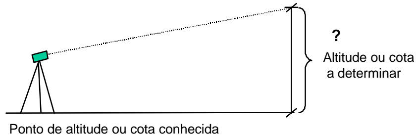
Figura 168 – Nivelamento Vante
