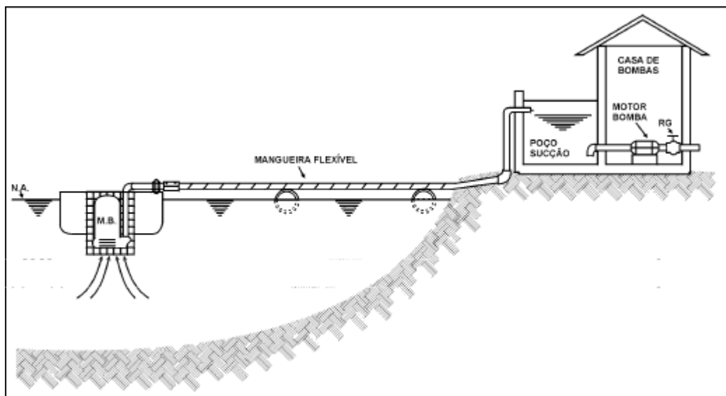
Figura 33 - Esquema de Tomada de Água Flutuante
