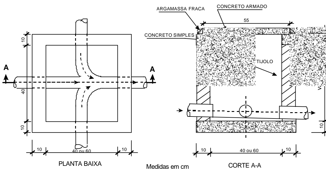
Figura 98 - Caixa de inspeção largura de 40 ou 60cm
