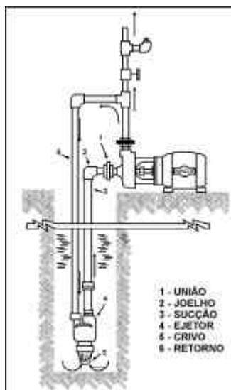
Figura 70 - Bomba Centrífuga com Ejetor
