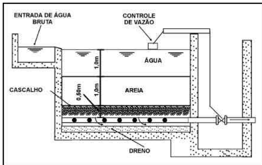
Figura 40 - Corte do Filtro Lento Detalhado
