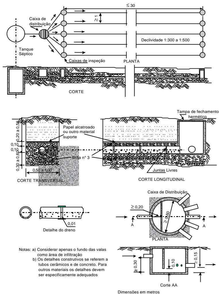
Figura 105 - Vala de Infiltração
