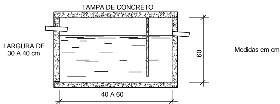
Figura 100 - Caixa de Gordura
