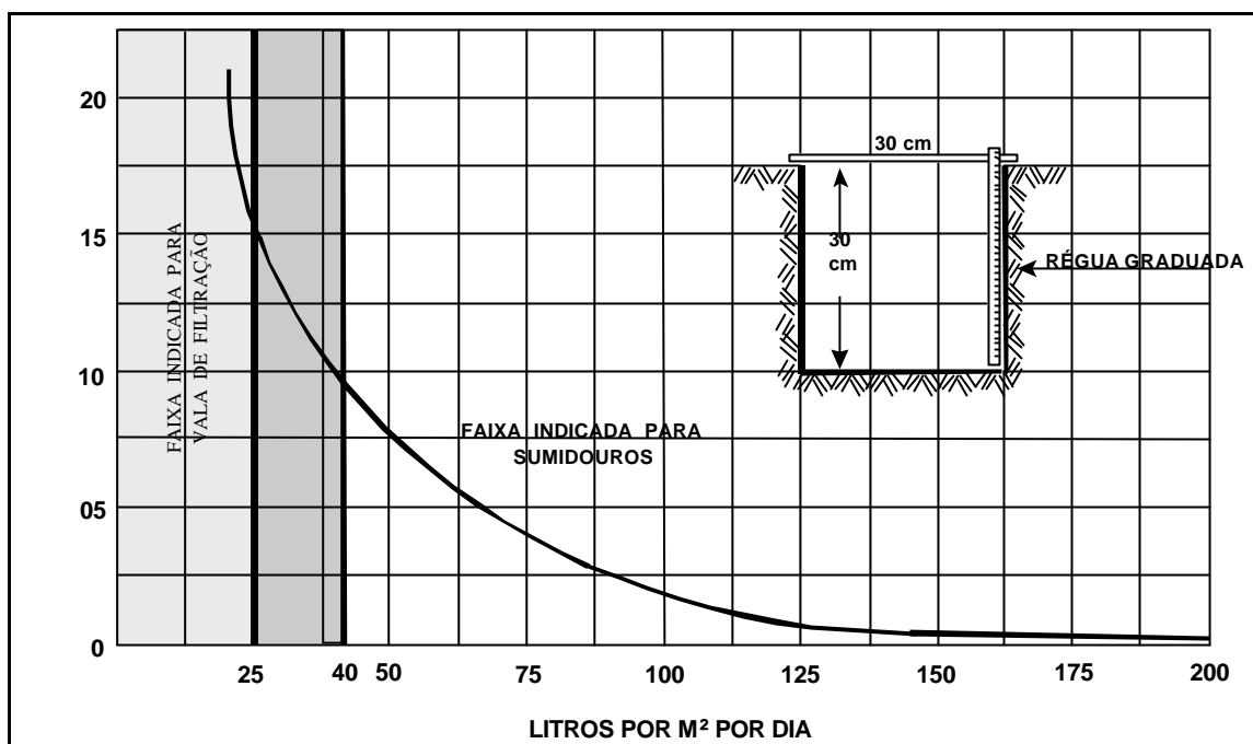
Figura 81 - Gráfico para Determinar Coeficiente de Percolação
