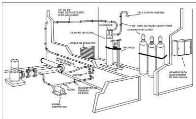
Figura 51 - Instalação Típica de Cloro Gasoso
