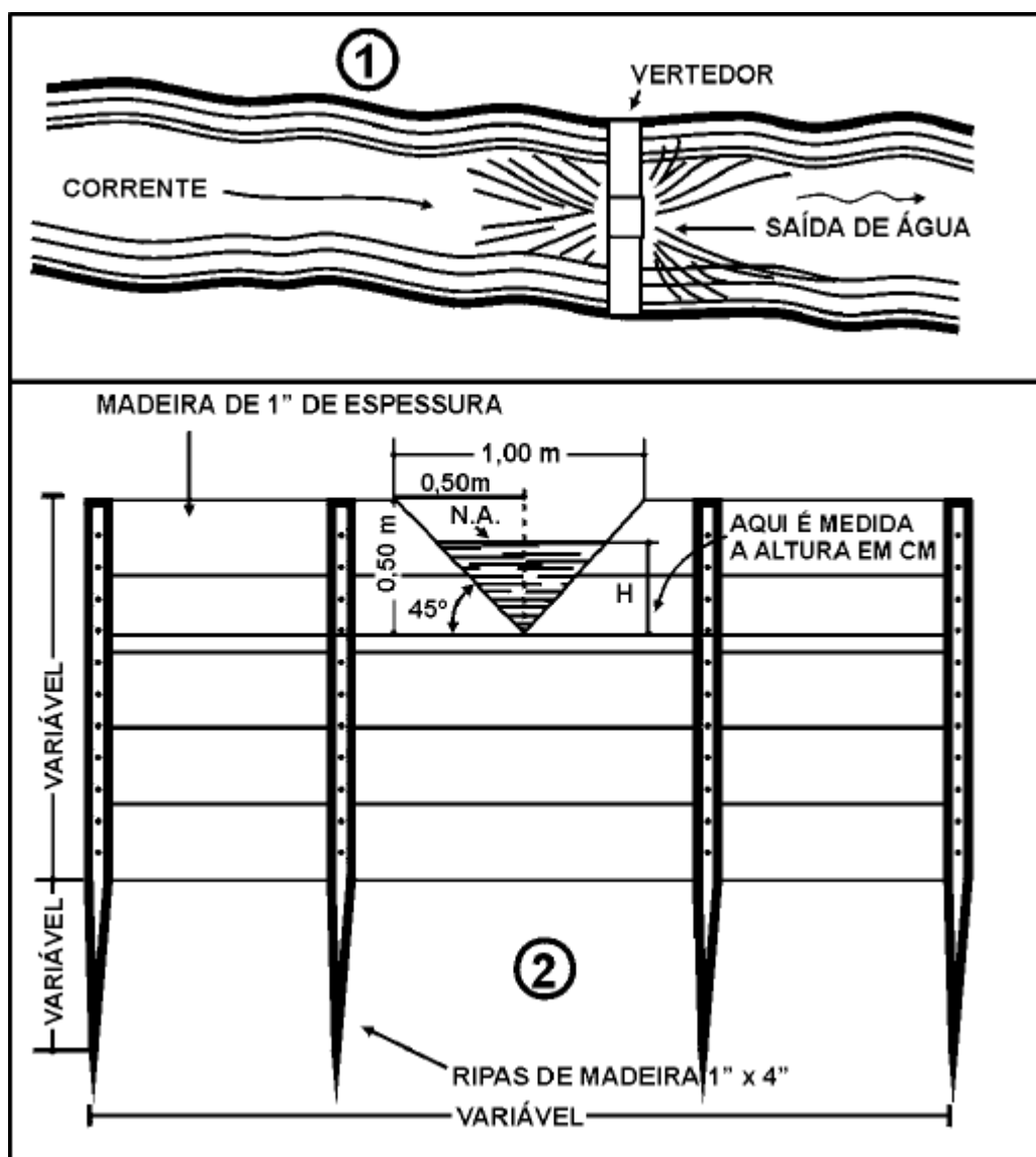
Figura 11 - Vertedouro de Madeira
