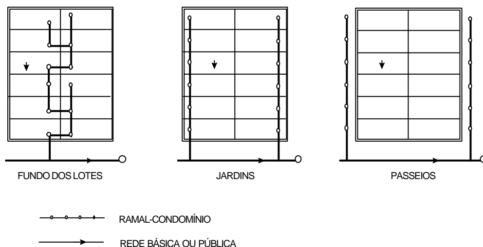
Figura 96 - Tipos Mais Comuns de Ramal Condominial
