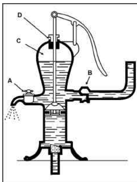
Figura 66 - Bomba Manual de Sucção e Recalque - Bomba de Êmbolo
