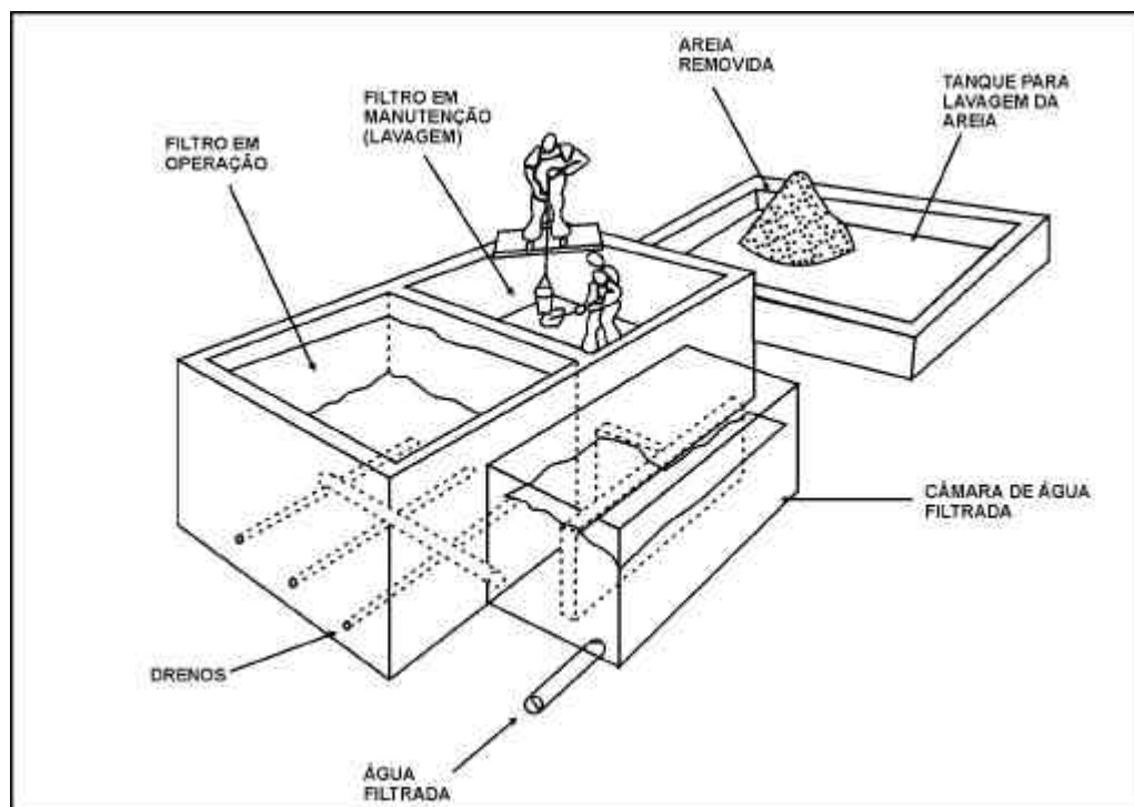
Figura 42 - Limpeza do Filtro Lento
