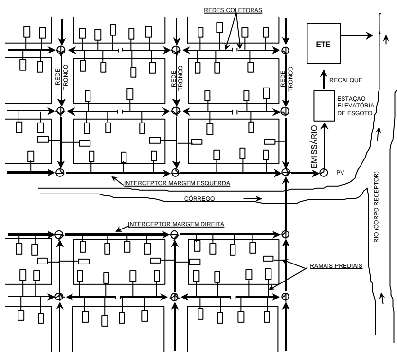
Figura 95 - Partes Constitutivas do Sistema Convencional
