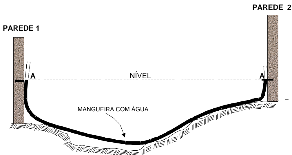
Figura 166 - Nivelamento do Terreno com Mangueira
