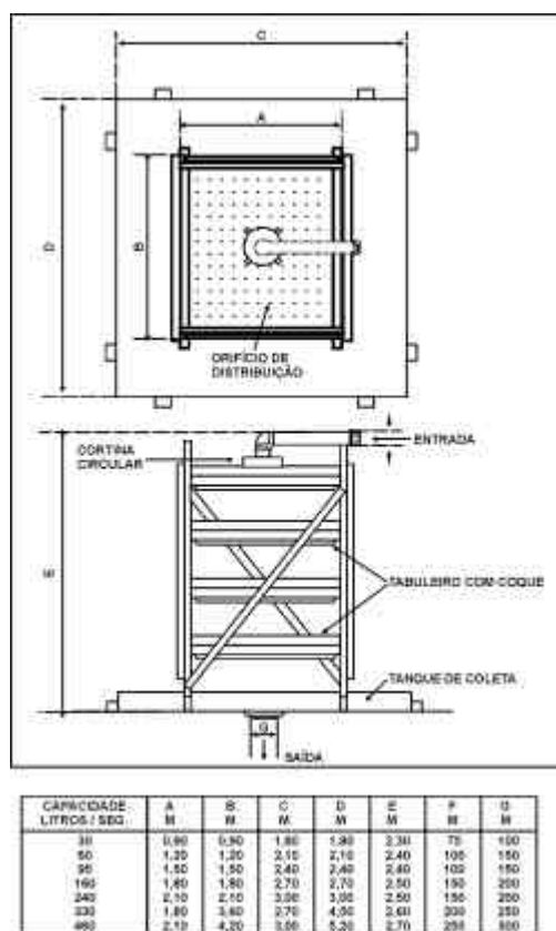
Figura 50 - Aerador de Tabuleiros ou Bandejas
