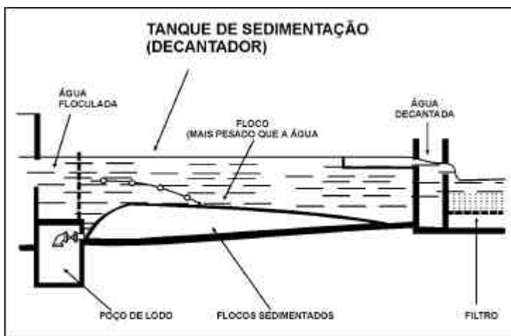
Figura 46 - Sedimentação
