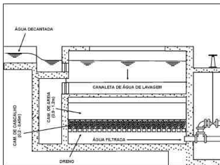
Figura 48 - Corte de Filtro Rápido Descendente
