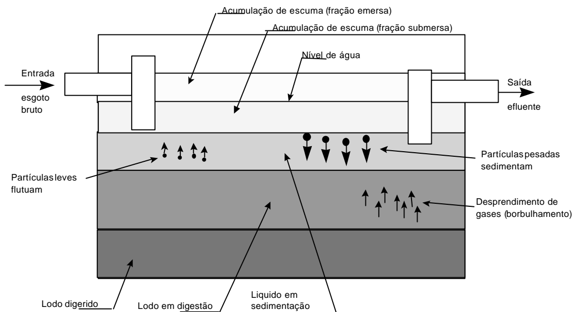
Figura 99 - Funcionamento Geral de um Tanque Séptico
