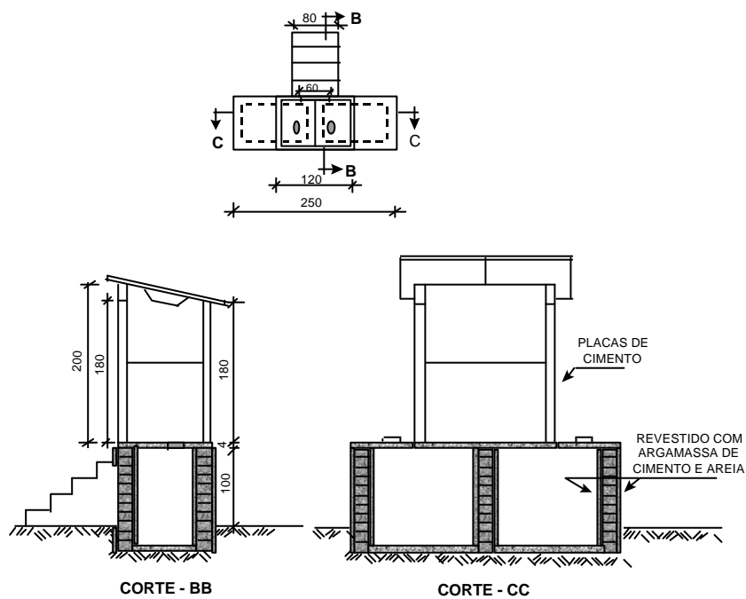
Figura 93 - Privada com Fossa de Fermentação Apoiada na Superfície do Solo
