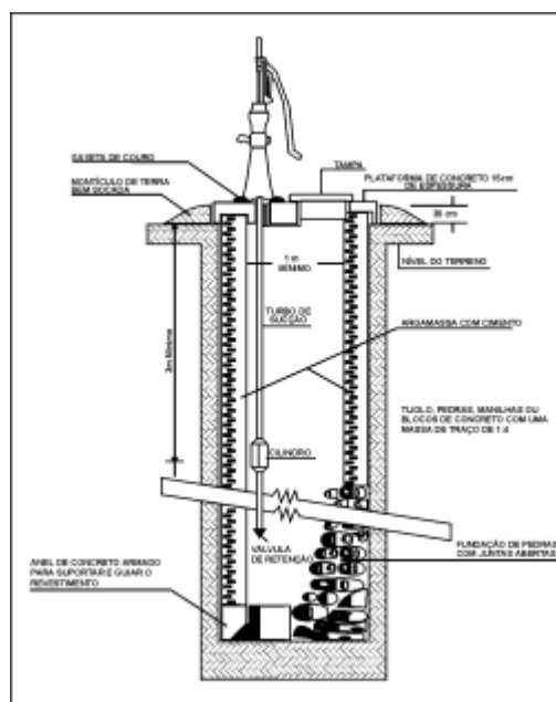
Figura 20 - Poço Construído Adequadamente
