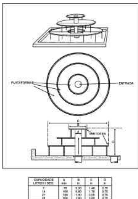
Figura 50 - Aerador de Tabuleiros ou Bandejas
