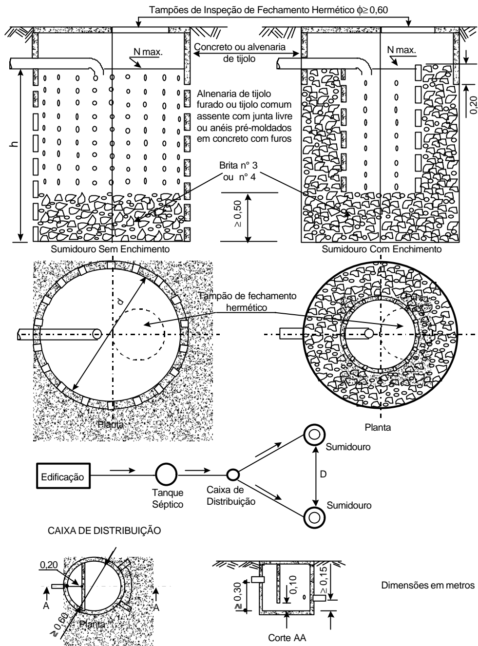
Figura 103 - Sumidouro Cilíndrico
