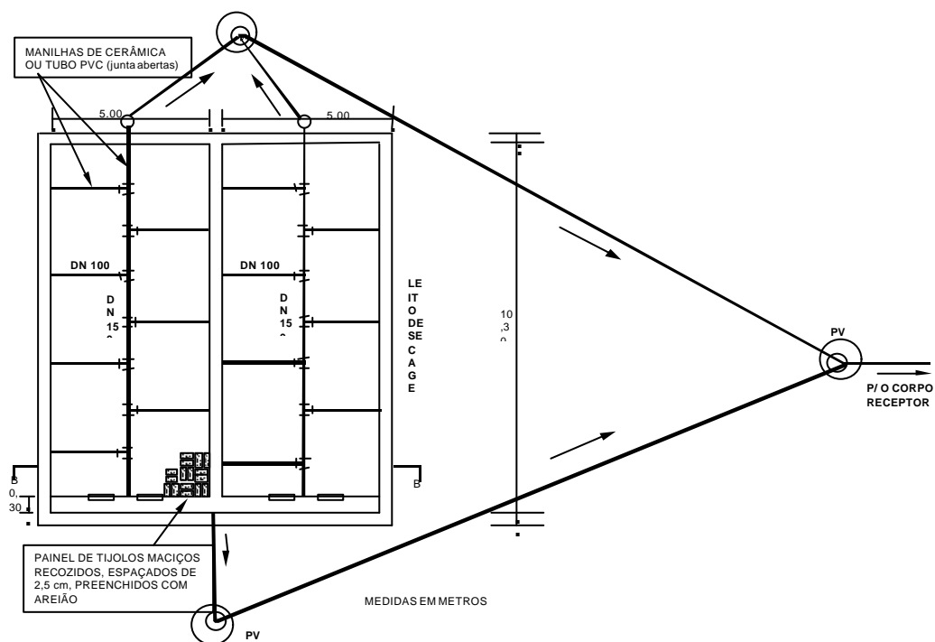
Figura 110 - Planta do Leito de Secagem
