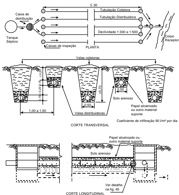
Figura 107 - Vala de Filtração em Terreno Arenoso
