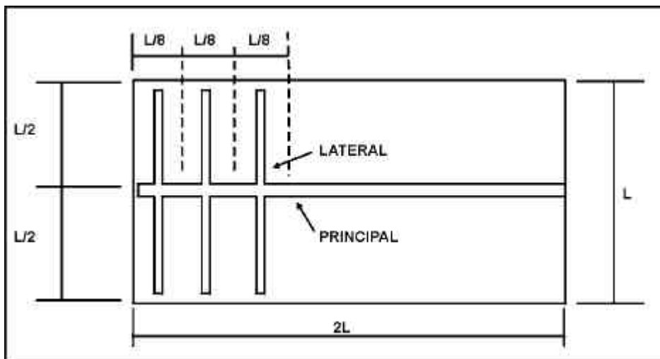
Figura 39 - Sistema de Drenagem
