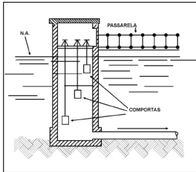
Figura 32 - Torre de Tomada
