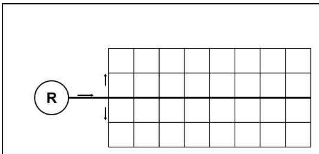
Figura 54 -Rede Malhada sem Anel
