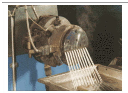
Foto 19 - Extrusora – Vista Frontal
