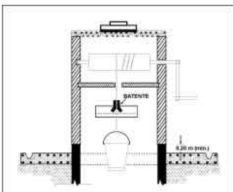
Figuras 64 e 65 – Sarilho com Proteção Sanitária
