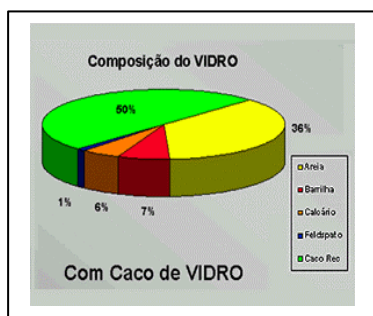
Figuras 114 - Composição do Vidro
