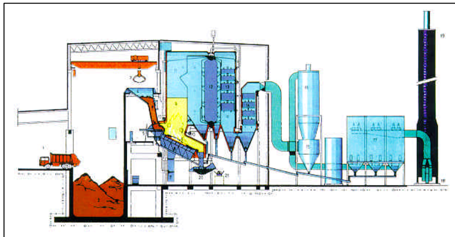
Figura 118 - Esquema de uma Usina de Incineração
