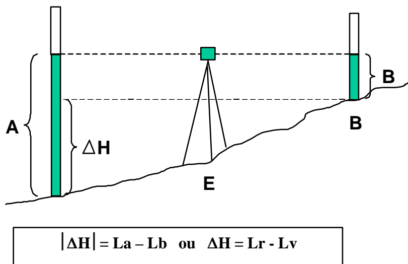
Figura 169 – Nivelamento Linear Simples I
