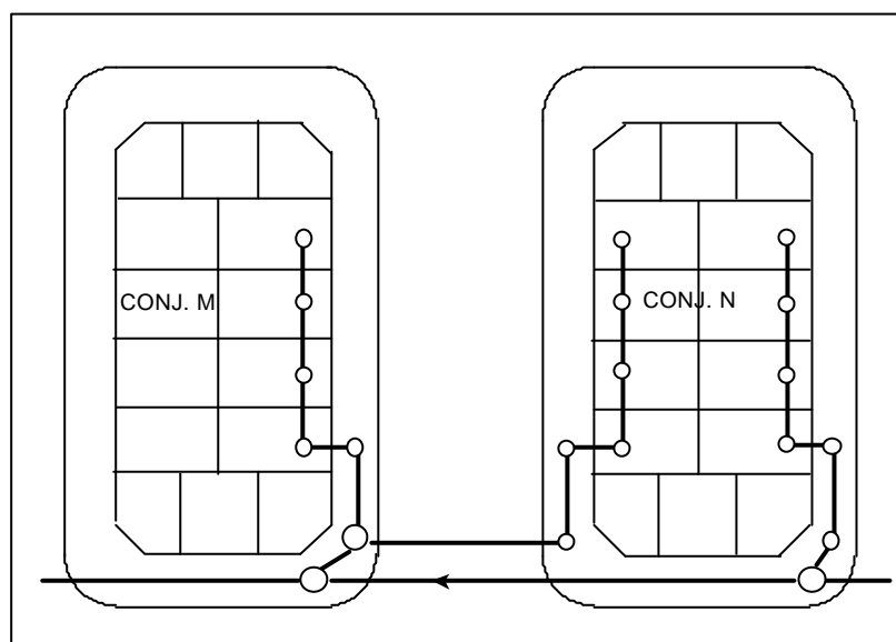
Figura 97 - Ligação de Dois Ramais de Conjuntos Diferentes Numa Mesma CI.
