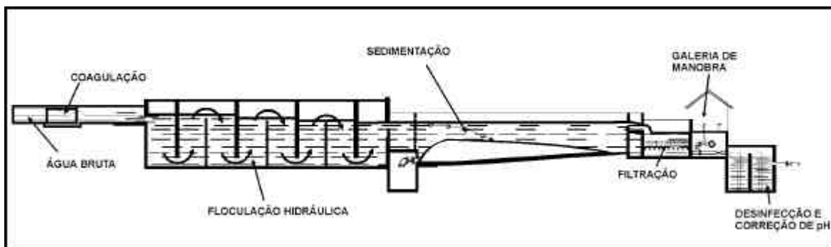
Figura 43 - Sequência do Tratamento Clássico ou Convencional
