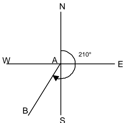
Figura 150 – Azimute de 210° à Direita
