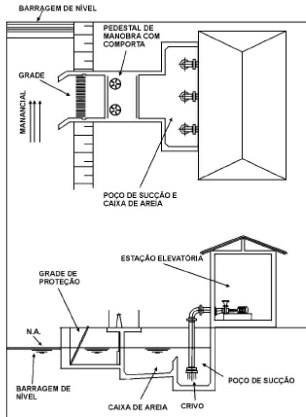
Figura 25 – Tomada de Água com Barragem de Nível
