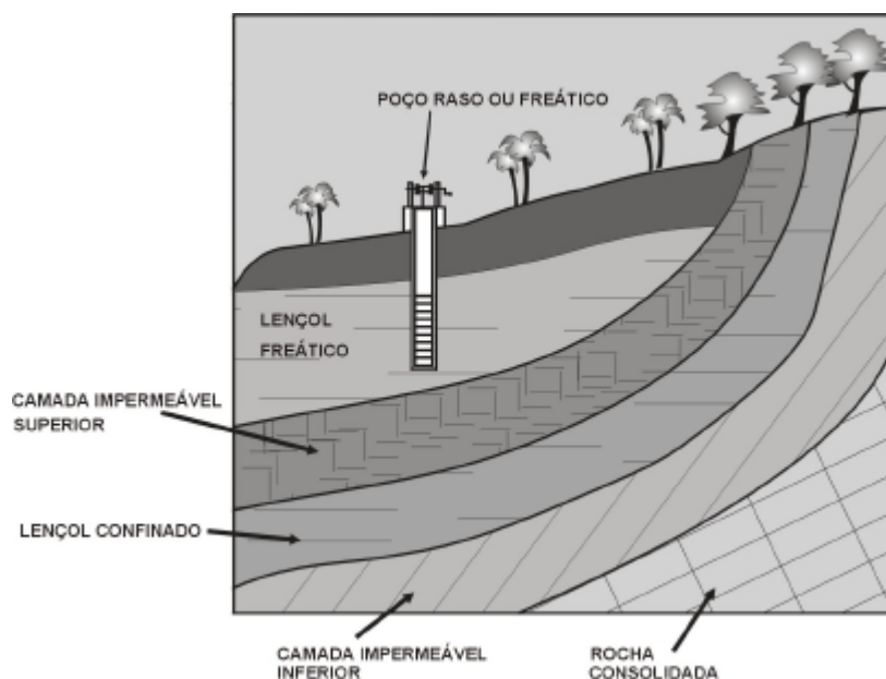
Figura 18 - Poço Raso
