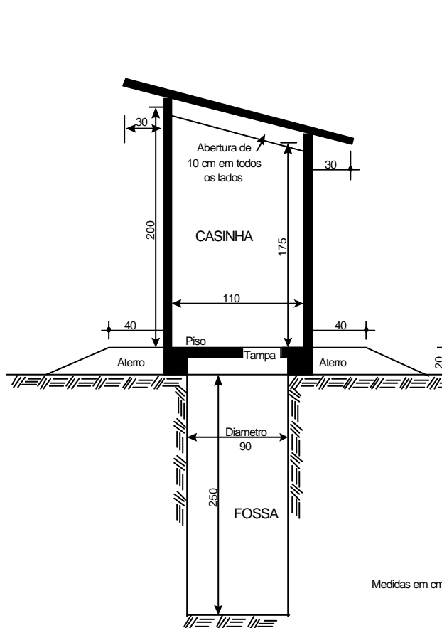
Figura 82 - Privada Convencional com Fossa Seca
