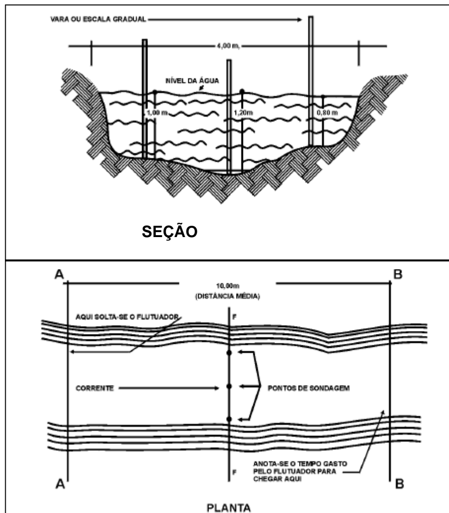
Figura 10 - Determinação da Seção Transversal
