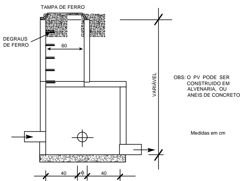
Figura 94 – Poço de Visita
