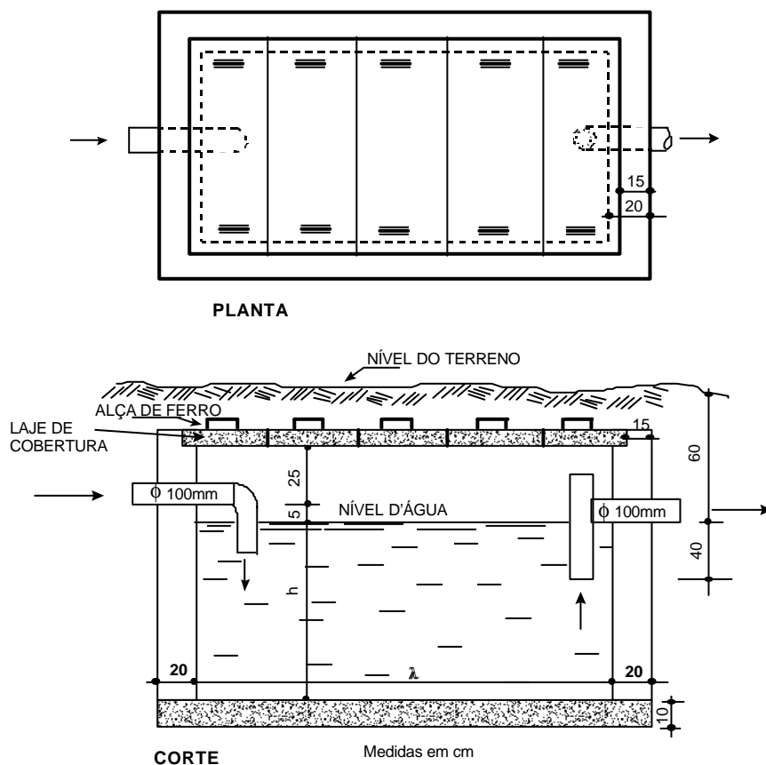
Figura 101 - Tanque Séptico Prismático
