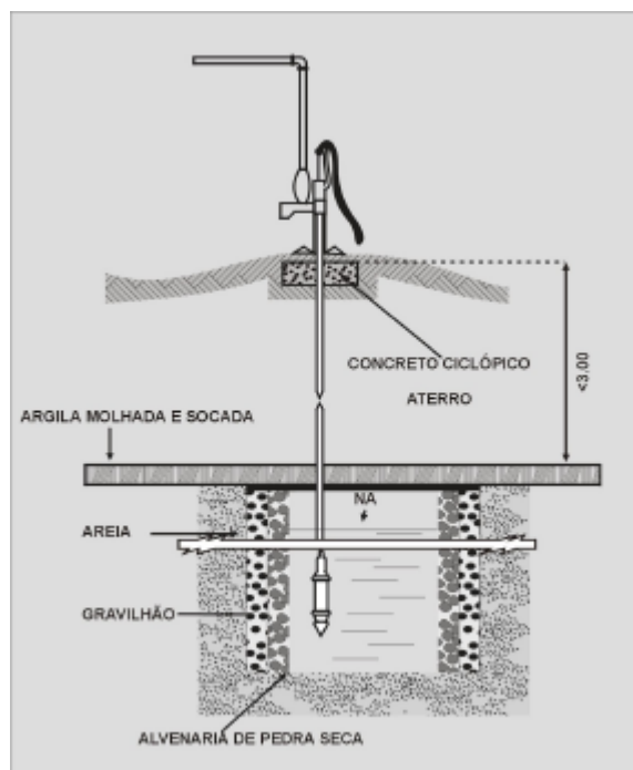
Figura 19 - Operação de Bomba Manual
