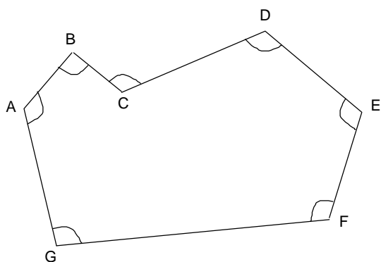
Figura 164 – Caminhamento Fechado
