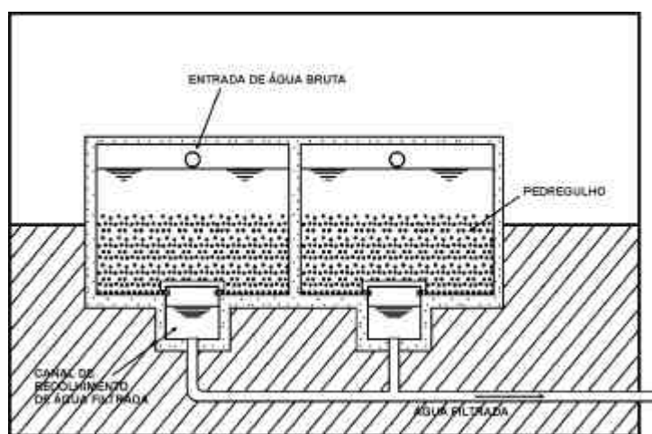
Figura 42 - Corte de um Pré-Filtro
