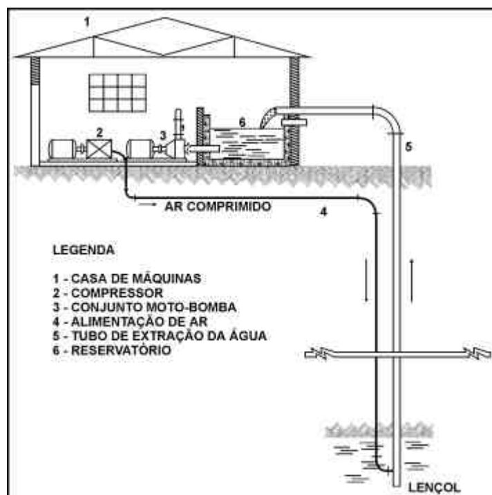
Figura 71 - Esquema de uma Instalação de Air-Lift
