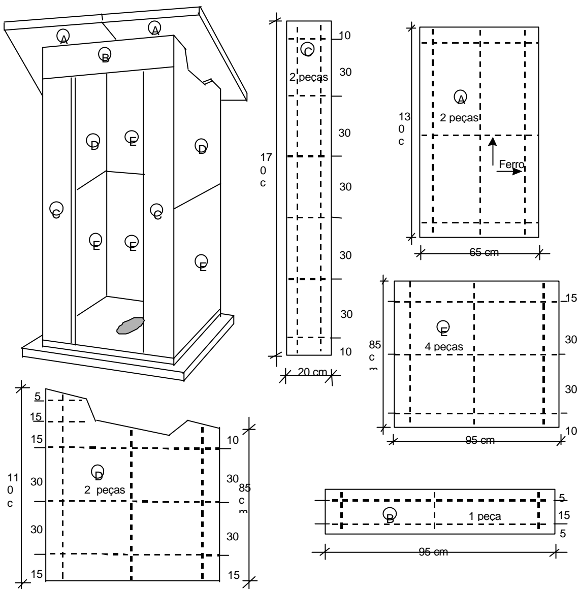
Figura 90 - Casinha Pré-Fabricada em Placas de Cimento
