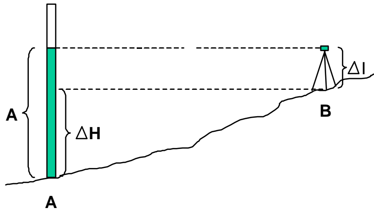
Figura 170 – Nivelamento Linear Simples II
