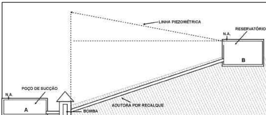
Figura 38 - Adutora por Recalque
