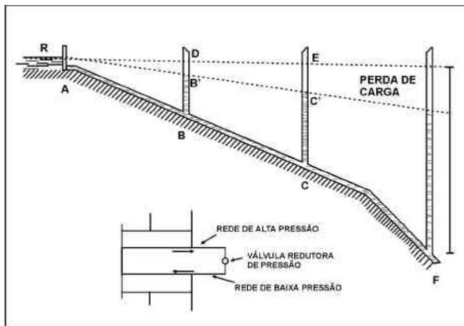
Figura 57 - Vasos Comunicantes Líquido em Regime de Escoamento
