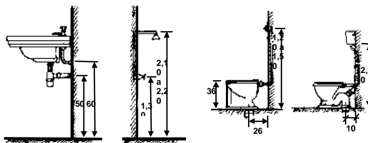
Figura 189 - Alturas das Saídas das Tubulações de Água
