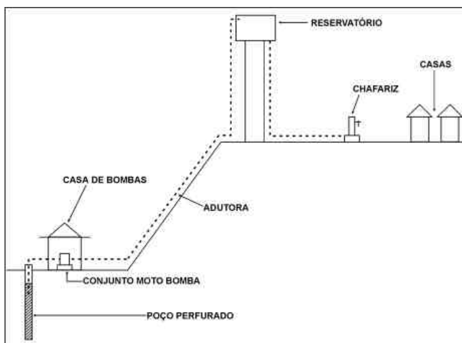
Figura 63 - Conjunto Poço, Elevatória, Adutora, Reservatório e Chafariz
