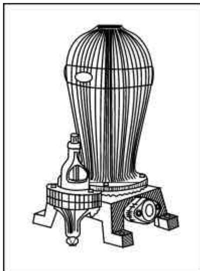
Figura 72 - Carneiro Hidráulico
