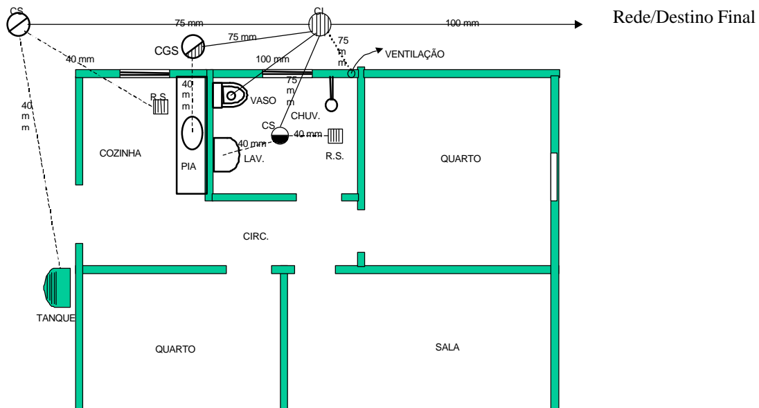
Figura 190 - Tubulações Indicadas para Cada Peça do Sistema de Esgotos Domiciliares
