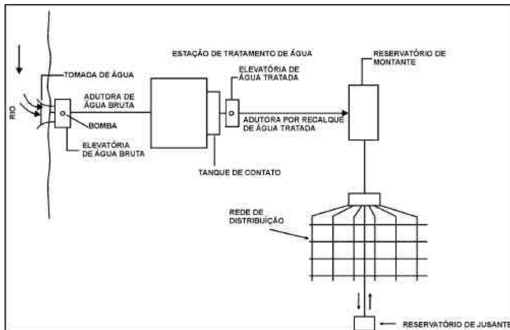
Figura 52 - Reservatório de Montante e Jusante
