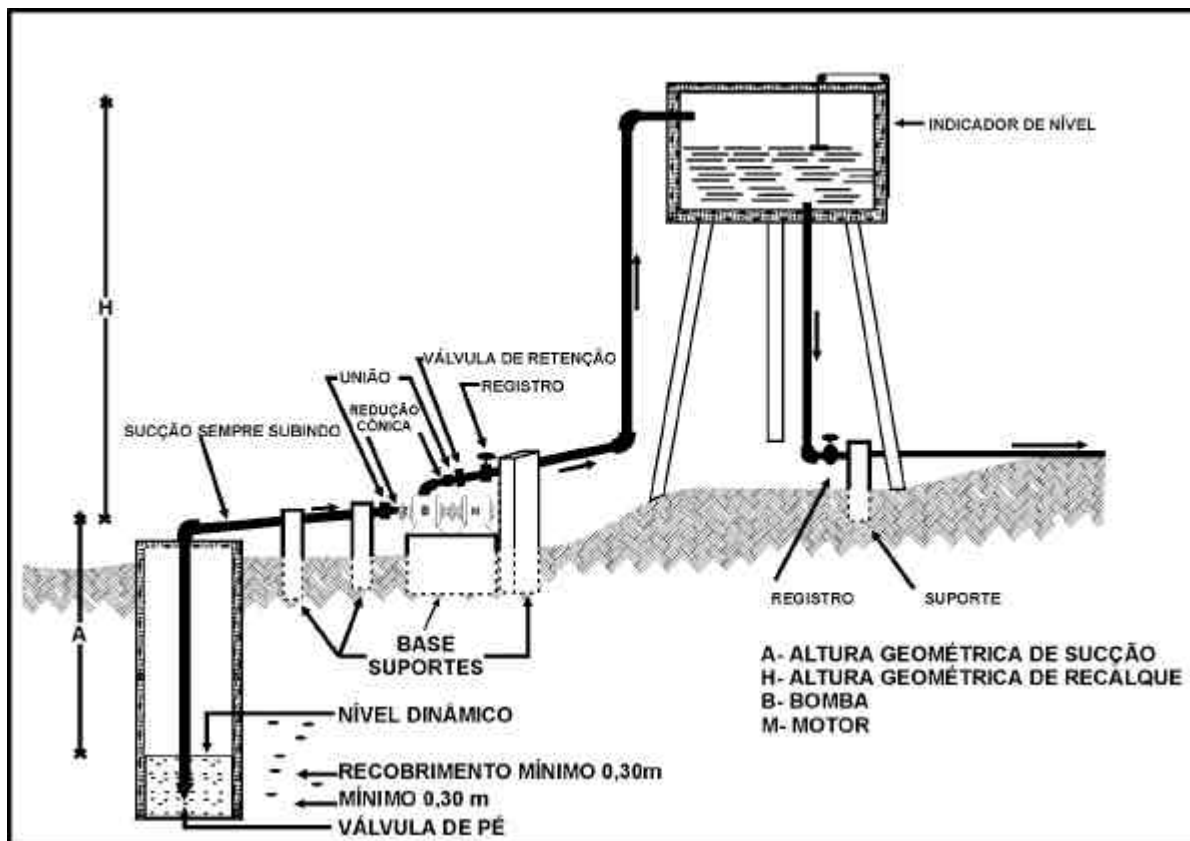
Figura 68 – Esquema de uma Instalação de Sucção e Recalque com Poço de Sucção
